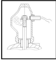
Виконання з індуктивним датчиком з сигналізацією
